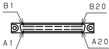
<コネクタピン配列図/CN1>
