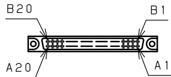
<コネクタピン配列図/CN2>
