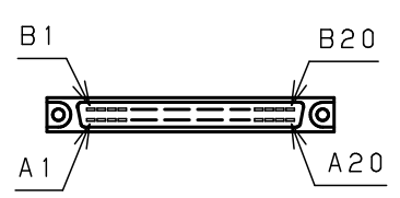
<コネクタピン配列図/CN1・CN2>
