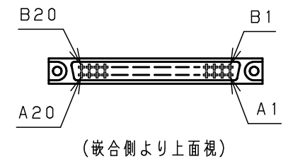
<コネクタピン配列図/CN3>
