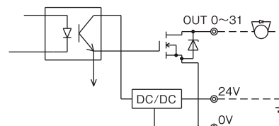
TKN-V32R(出力回路)
