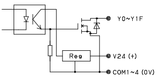
<出力回路>
