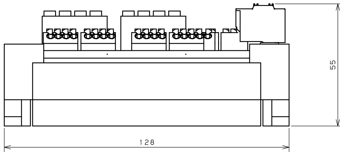
通信コネクタ 2EDGKDH-5, 08-6P (DEGSON)
