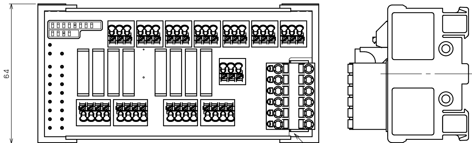
通信コネクタ 2EDGKDH-5, 08-6P (DEGSON)
