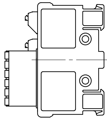
電源・通信コネクタ 2EDGKDH-5, 08-6P (DEGSON)
