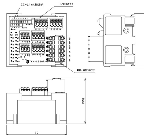
《外形図》
