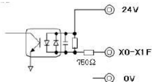
《外部接続例》
