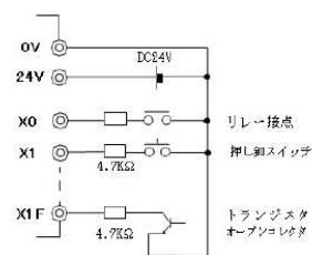
《外部接続例》
