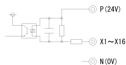
《外部接続例》
