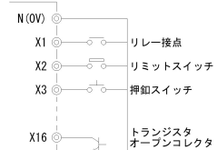
《外部接続例》
