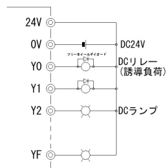
《外部接続例》
