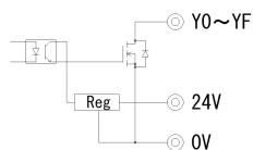
《外部接続例》
