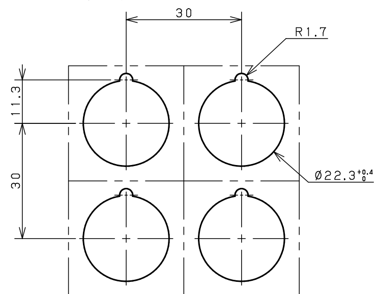
パネルカット寸法
