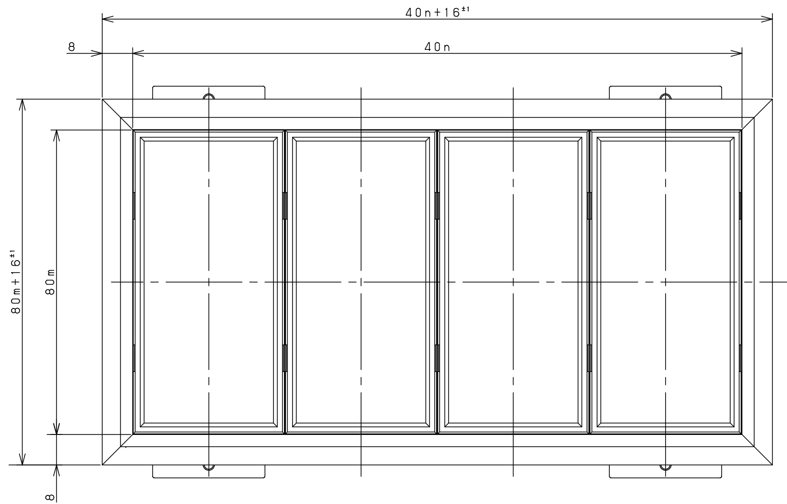
パネルカット寸法
