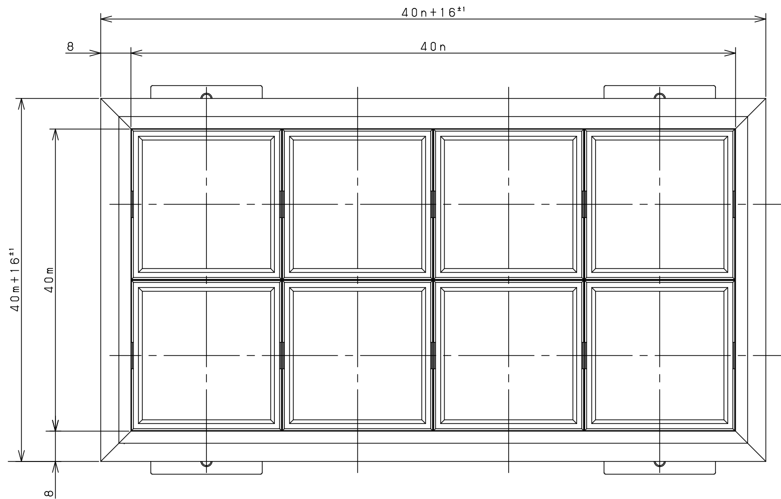
ハ° ネルカット寸法
