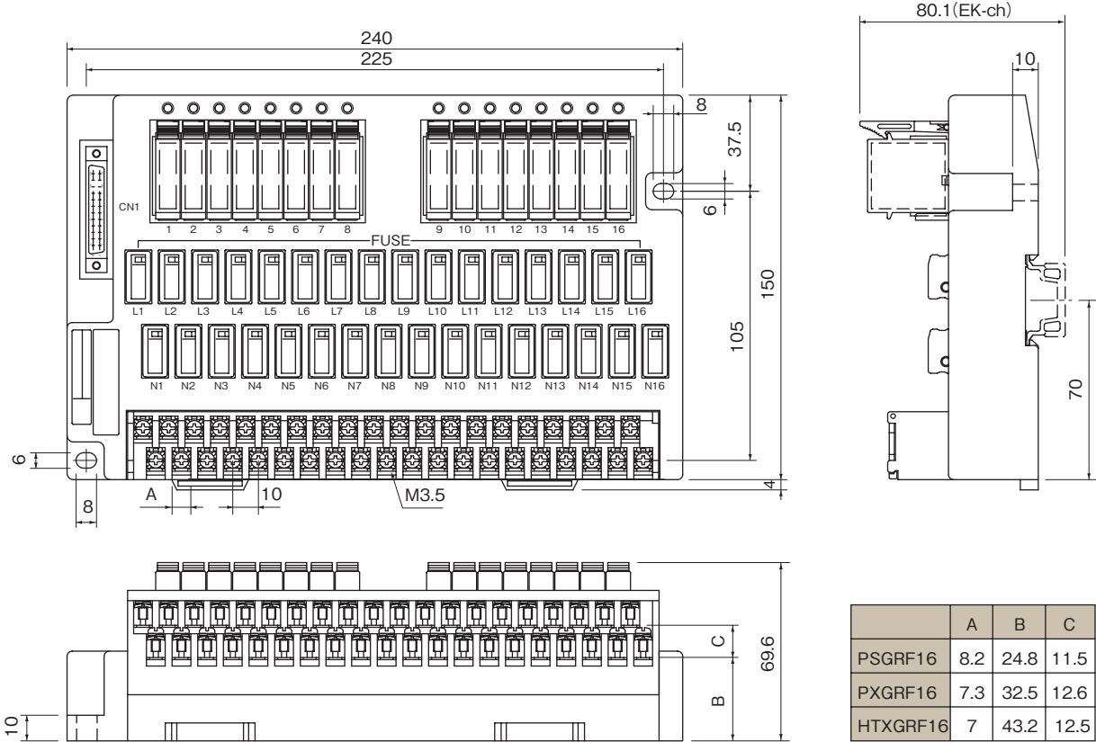
外形寸法図
