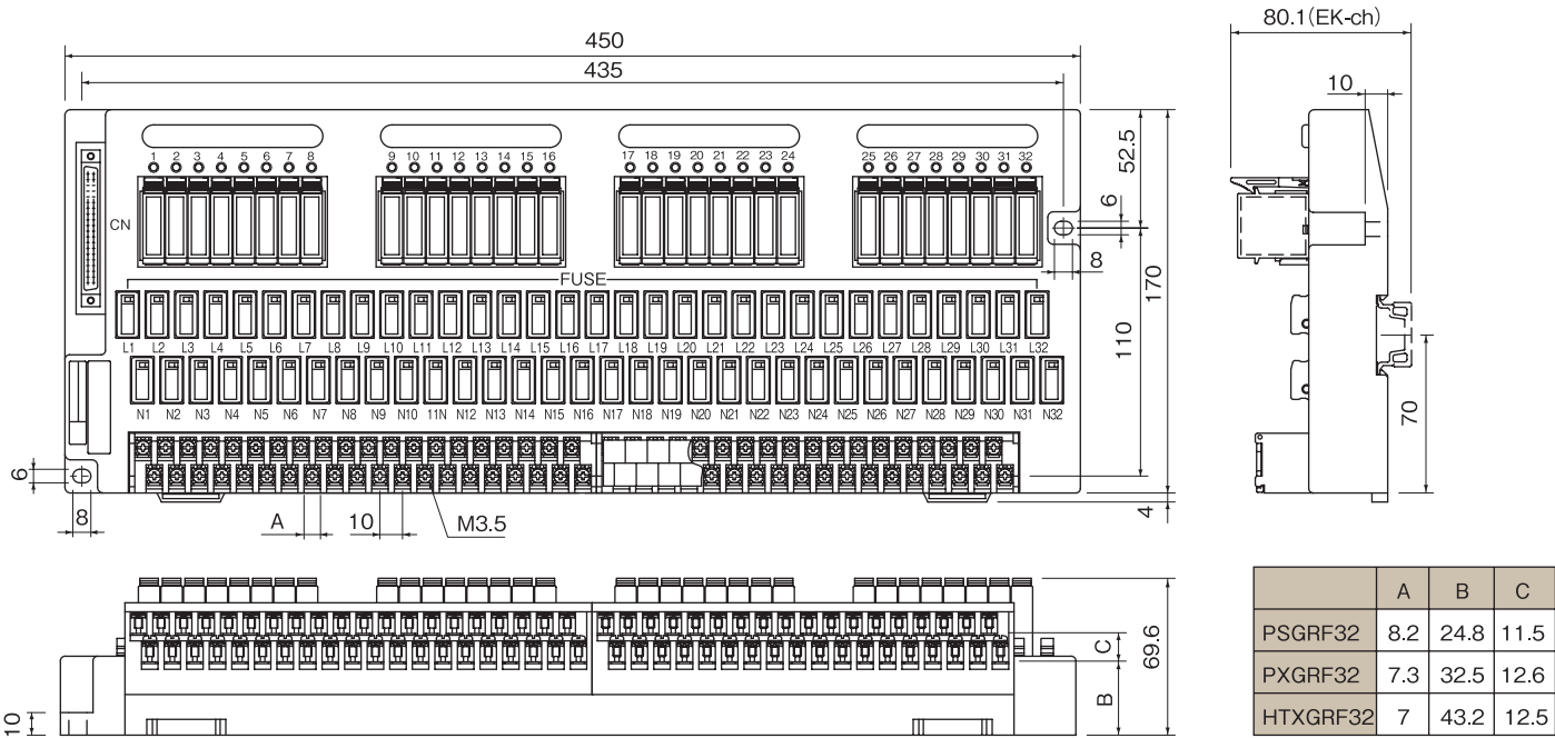
外形寸法図
