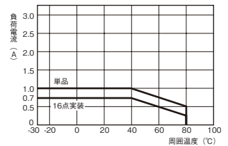
G3TA-OD201S
