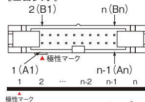
極性マーク
